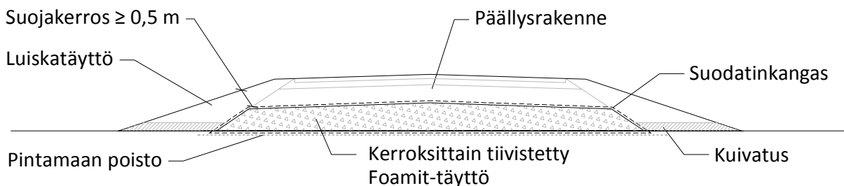
Kuva 3.1. Tie- tai katupenkereen osittaiskevennyksen Foamitilla.
