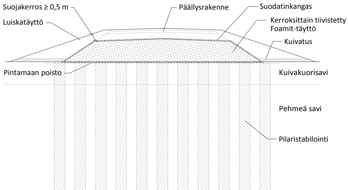
Kuva 3.2. Foamit korkean penkereen kevennä pengertäytönä pilaristabiloidun pohjamaan päällä. Kevennystä käyttäen on mahdollista harventaa pilariväliä, käyttää alemmaa pilarilujutta tai toteuttaa syvästabiloinnin varaisesti tavanomaista korkeampia penkereitä.
