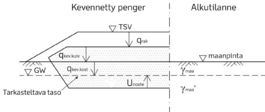
Kuva 3. Kevennysrakenteen nostemitoitus, merkinnät.
