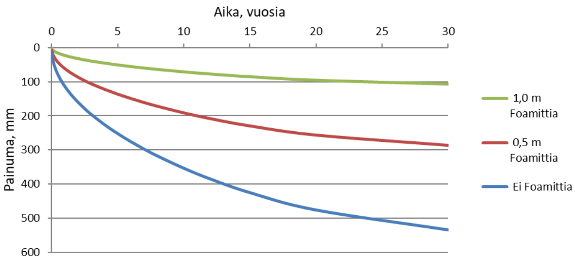
Kuva 3.5. Rakenteen kuormittaman pohjamaan aikapainumakuvaaja tapauksessa, jossa rakenteen alapuolella on savea 10 m kerros, saven vesipitoisuus 100 %, penkereen yläpinta 0,5 m alkuperäisen maapinnan yläpuolella, kevennys Foamitia, päälysrakennekerrokset 0,4 m Foamitin päällä.
