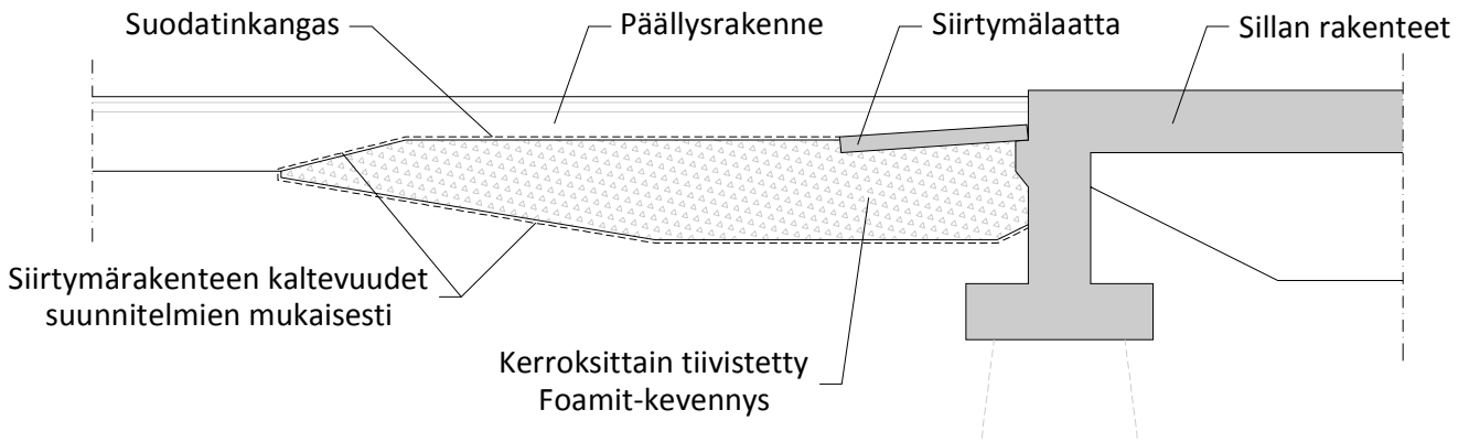
Kuva 3.4. Foamitista rakennettu sillan tulopenkereen kevennys- ja siirtymärakenne.
